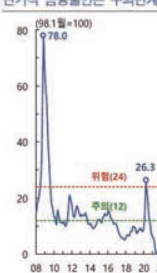
[그림 1] 금융불안지수(FSI) 1)
