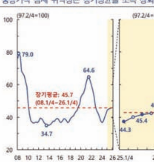
[그림 2] 금융취약성지수(FVI) 1)
