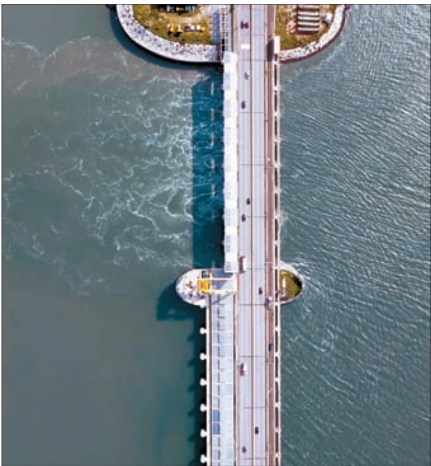
경기 안산 시화호조력발전소. 서해와 시화호의 낙차를 이용해 전기를 생산한다. 아래 사진은 1994년 방조제가 완공된 후 죽음의 호수로 변한 모습. 푸른 바다와 달리 시화호는 오페수 유입으로 검게 오염돼 있다. [사진 한국수자원공사]
