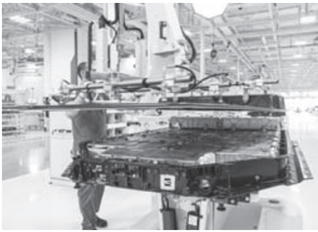
(왼쪽부터) 페라리 본사 공장에서 작업자가 전기차 배터리 팩을 조립하고 있다. 페라리가 공개한 첫 전기차 플랫폼 ‘일렉트리카’. [페라리 제공]
